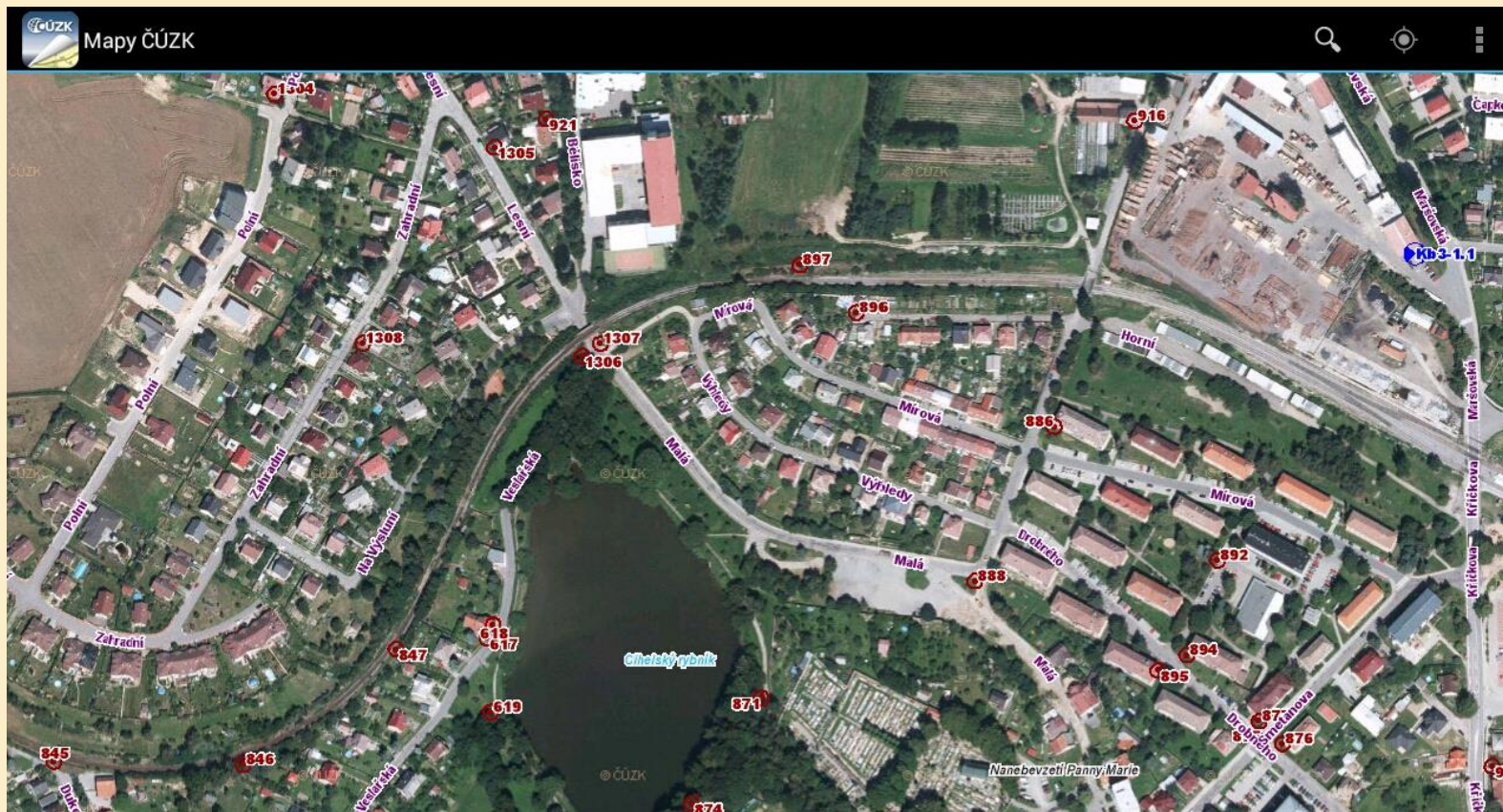
Obr. 7: Mapa bodových polí je doplněna o vybrané body s přesně určenou polohou a nadmořskou výškou. Modře jsou výškopisné (nivelační body) s přesně zaměřenou nadmořskou výškou, červeně polohové body s přesně zaměřenou zeměpisnou polohou.
